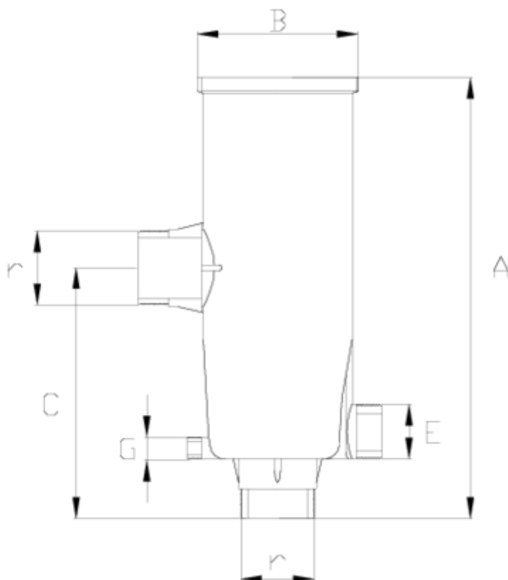
ITEM 701 | CUERPO FILTRO SALIDA ROSCADA "BSP" PPFV
